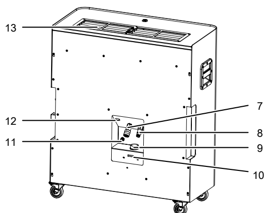
AC 7000 - inomhusenhet
