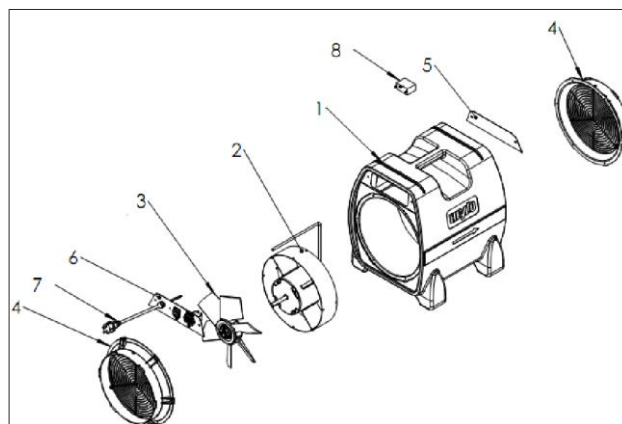
Abb. 2: Ersatzteile PV 3000
