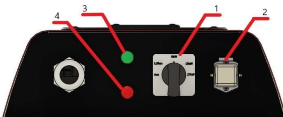
Abb. 3: Bedien/Anzeigeelemente
